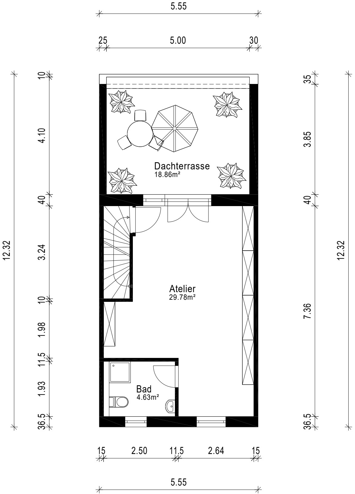
Dachgeschoss
