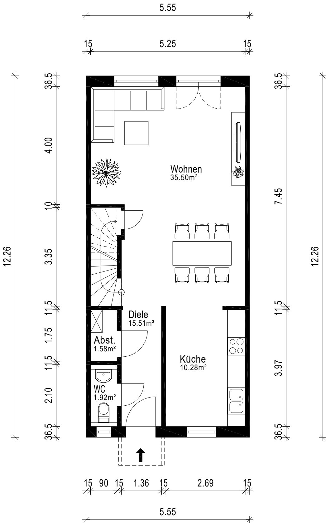
Erdgeschoss
